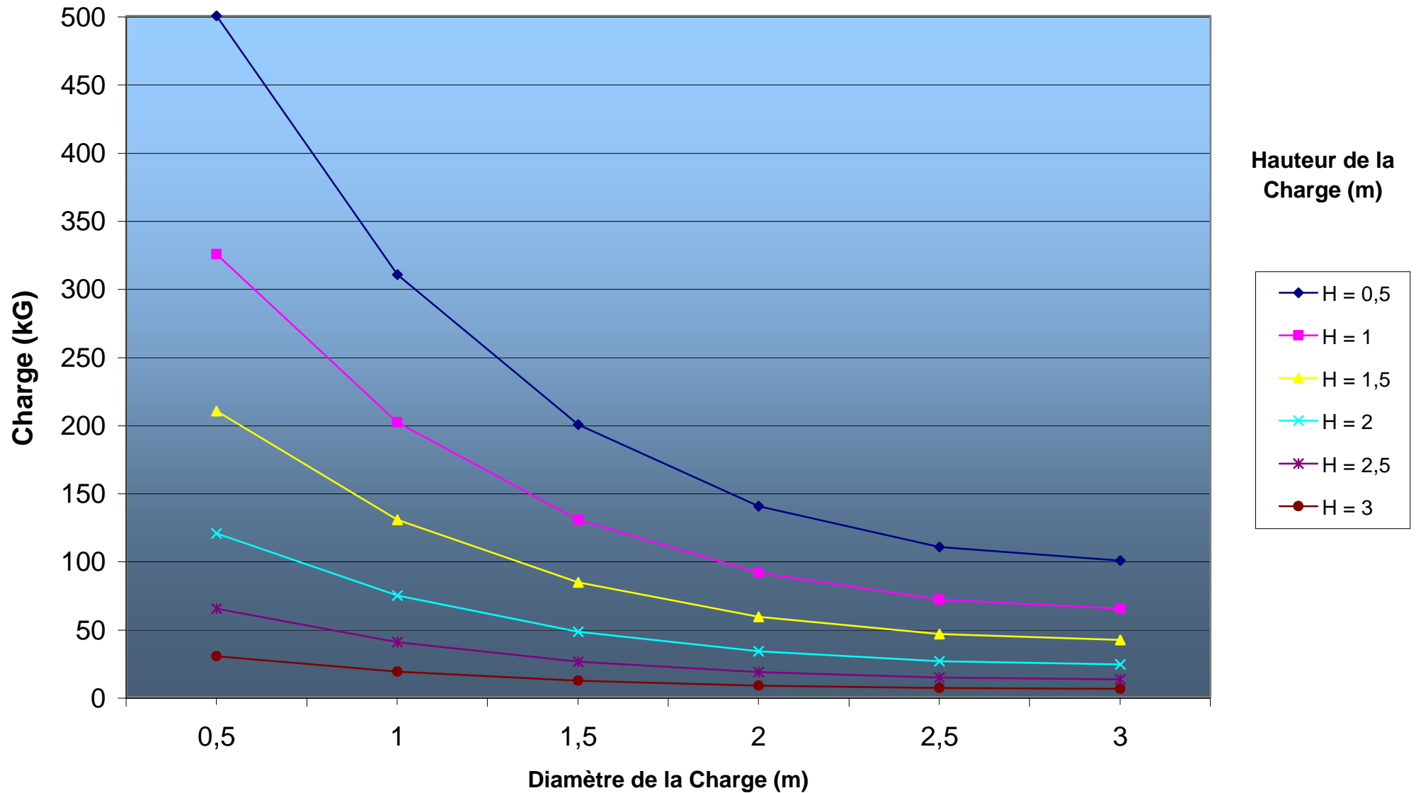
Podium tournant Gammes ATS et ATD (AT./B/1/2/3)
